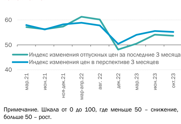
Рис. 3. Как изменились и как изменятся отпускные цены вашей компании?
