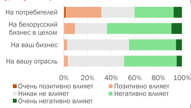
Рис. 1. Влияние ситуации с регулированием цен (декабрь 2022)
